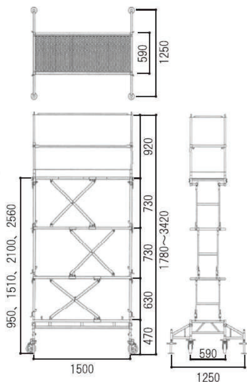
外形図(25型・単位:mm)
