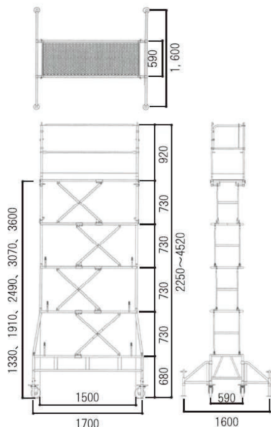
外形図(36型・単位:mm)
